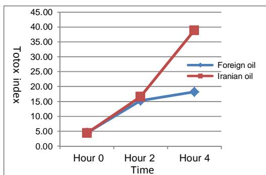
شکل ۴ مقایسه تغییرات اندیس توتوکس طی فرایند حرارتی
